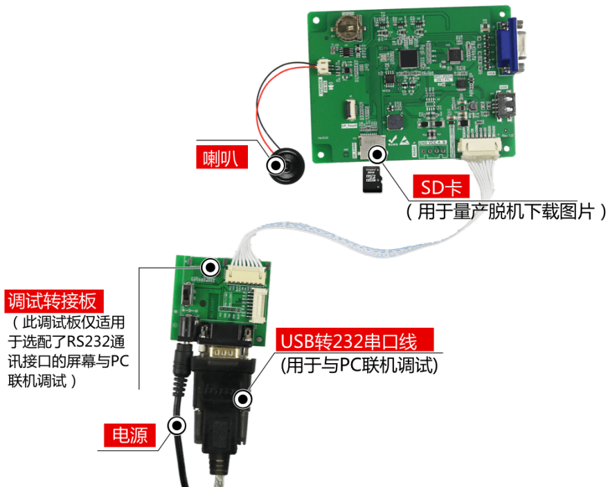
图 1-3 硬件调试图
